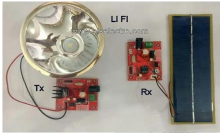
Fig. 2: Li-Fi module
